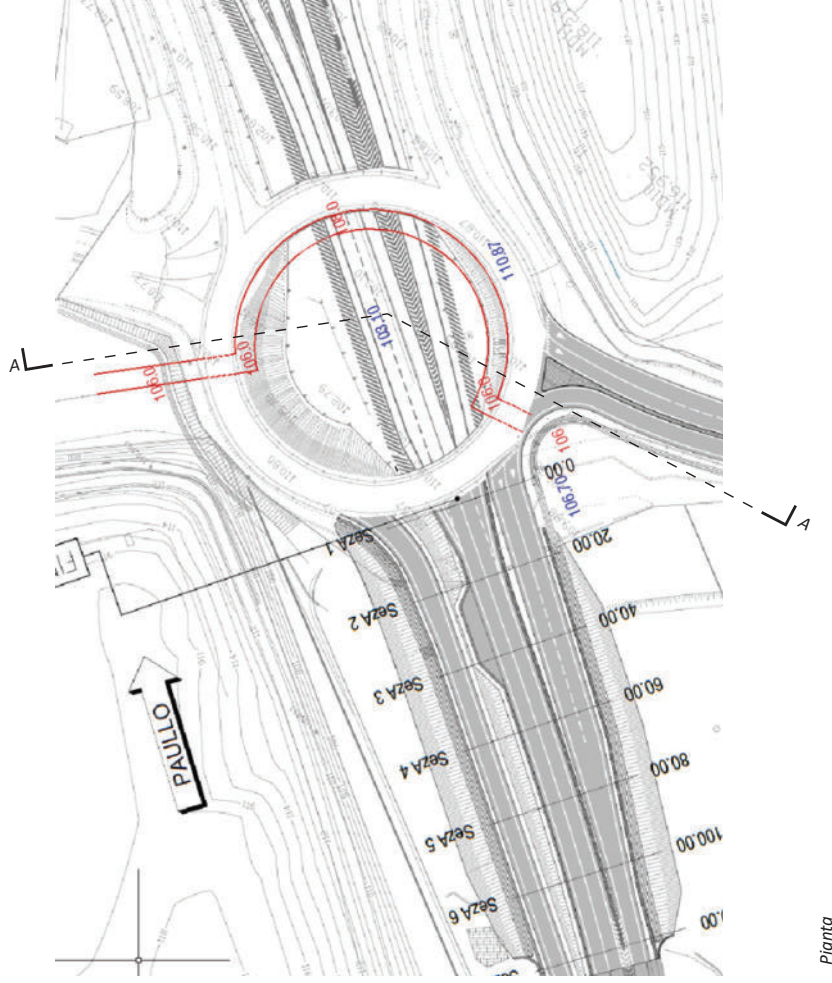
Fig. 2 Studio del collegamento ciclabile Arena-M3 Rogoredo in corrispondenza della rotonda SS Paullese (pianta e sezione trasversale)
